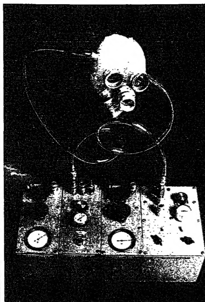
القلب الاصطناعي «فيليق» مع كامل اتابيب الضخ النموذج الجديد
